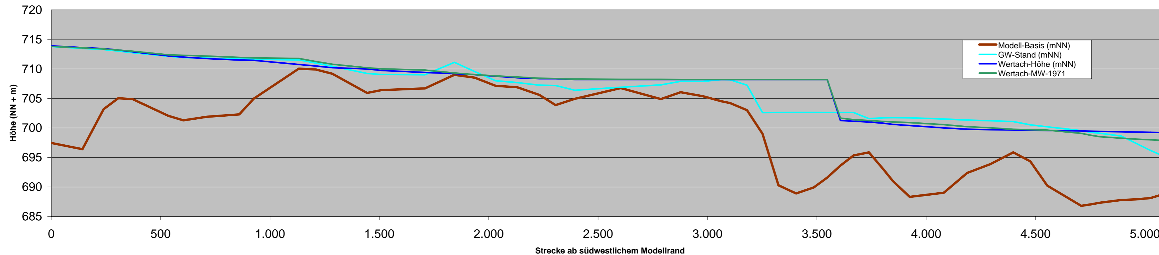
Wertachprofil von Modellrand zu Modellrand - Rechenfall 1
