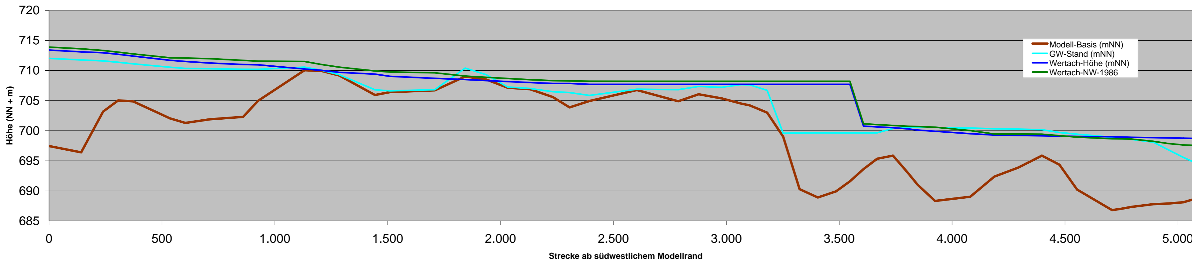
Wertachprofil von Modellrand zu Modellrand - Rechenfall 5
