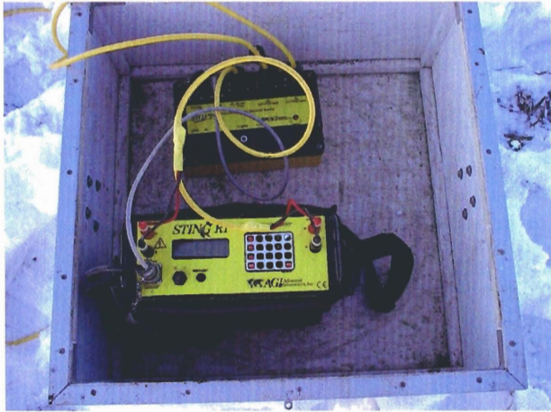
Foto 1 : Eingesetztes Messsystem Sting / Swift der Firma AGI Inc. ( USA)
